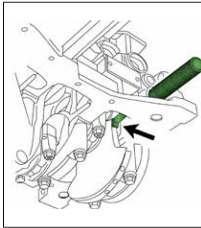
9B krukas timing gereedschap
